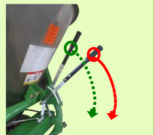
คันโยกปรับปุ๋ยและทิศทางการหวาน
